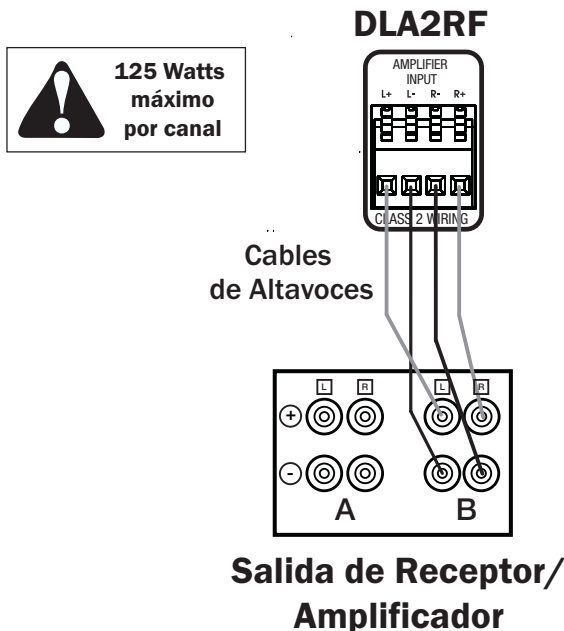
Dibujo 3-1: Salida de Receptor/Amplificador a la Entrada de Amplificador del DLA2RF
